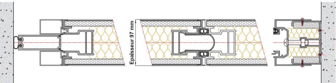
Montant Télescopique
